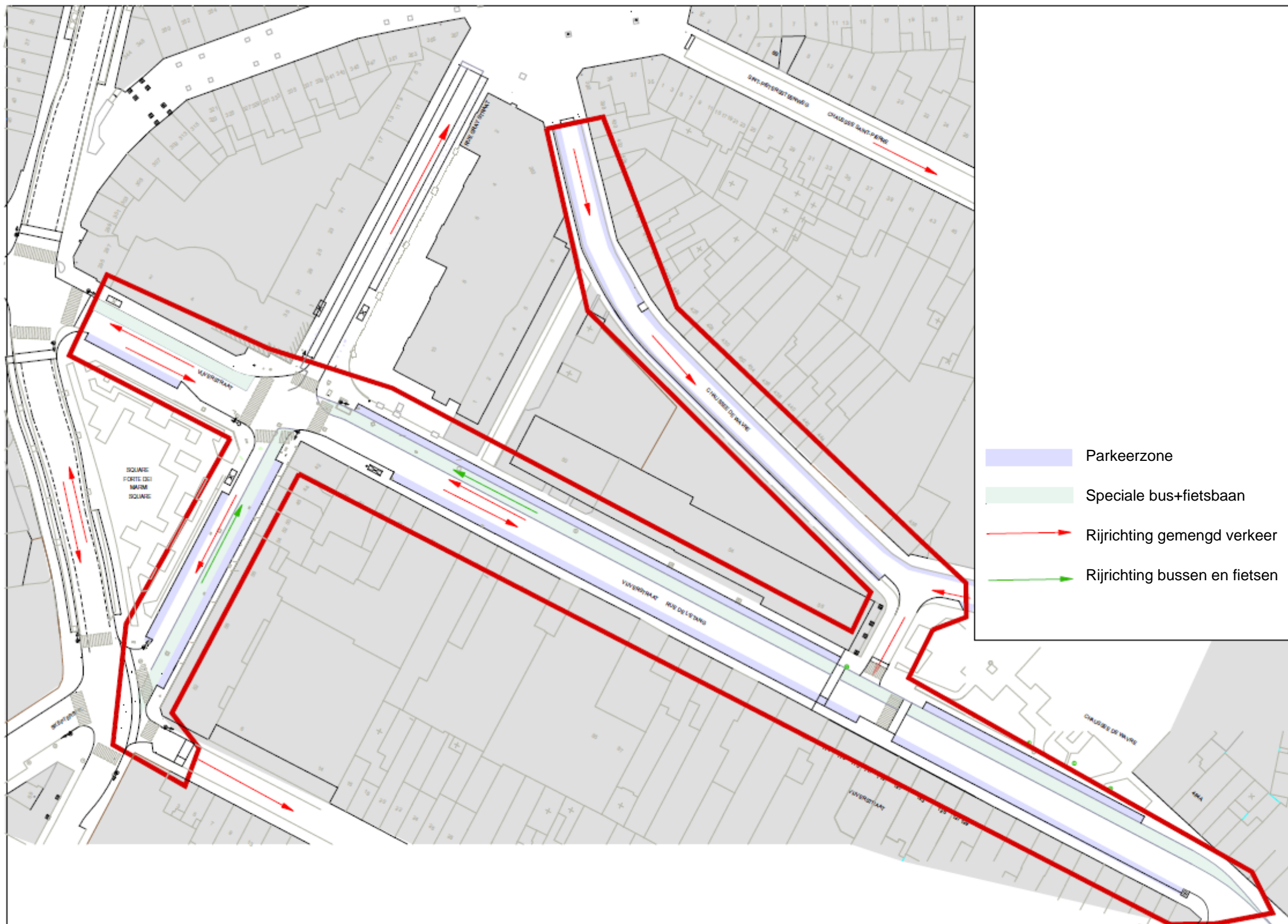
Aanlegprincipe Vijverstraat: Ontwerp Gemeente /Planeco
